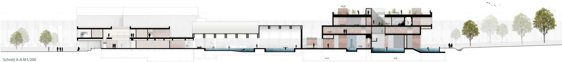
Schnitt A-A M1/200
